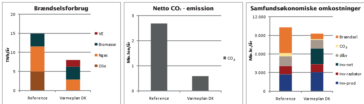
Figur 1: Varmeplan Danmarks udbygningsplan frem til 2020 sammenlignet med at beholde de nuværende individuelle olie-, gas- og biomassefyr. Udbygningsplanen omfatter 24 % af varmemarkedet. Og der er forudsat varmebesparelser svarende til en reduktion i rumvarmebehovet på 25 % i såvel referencen som i Varmeplan DK alternativet.
